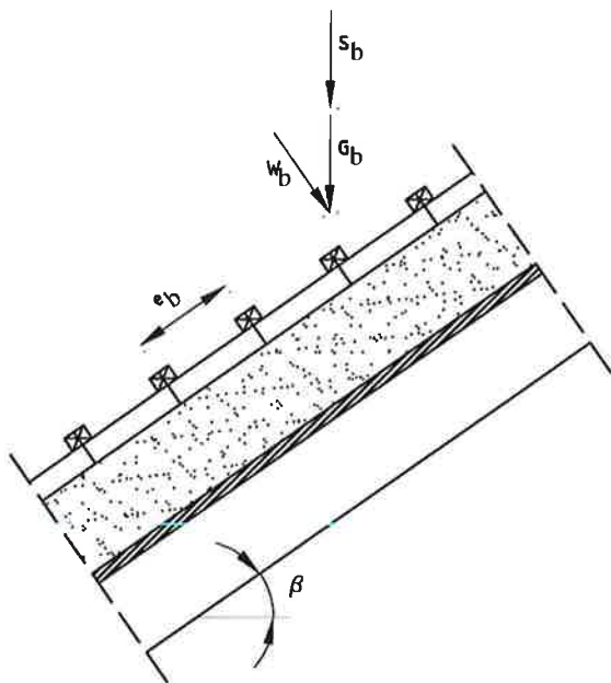
Abbildung 3.2: Einzellasten F_b rechtwinklig zu den Konterlatten
