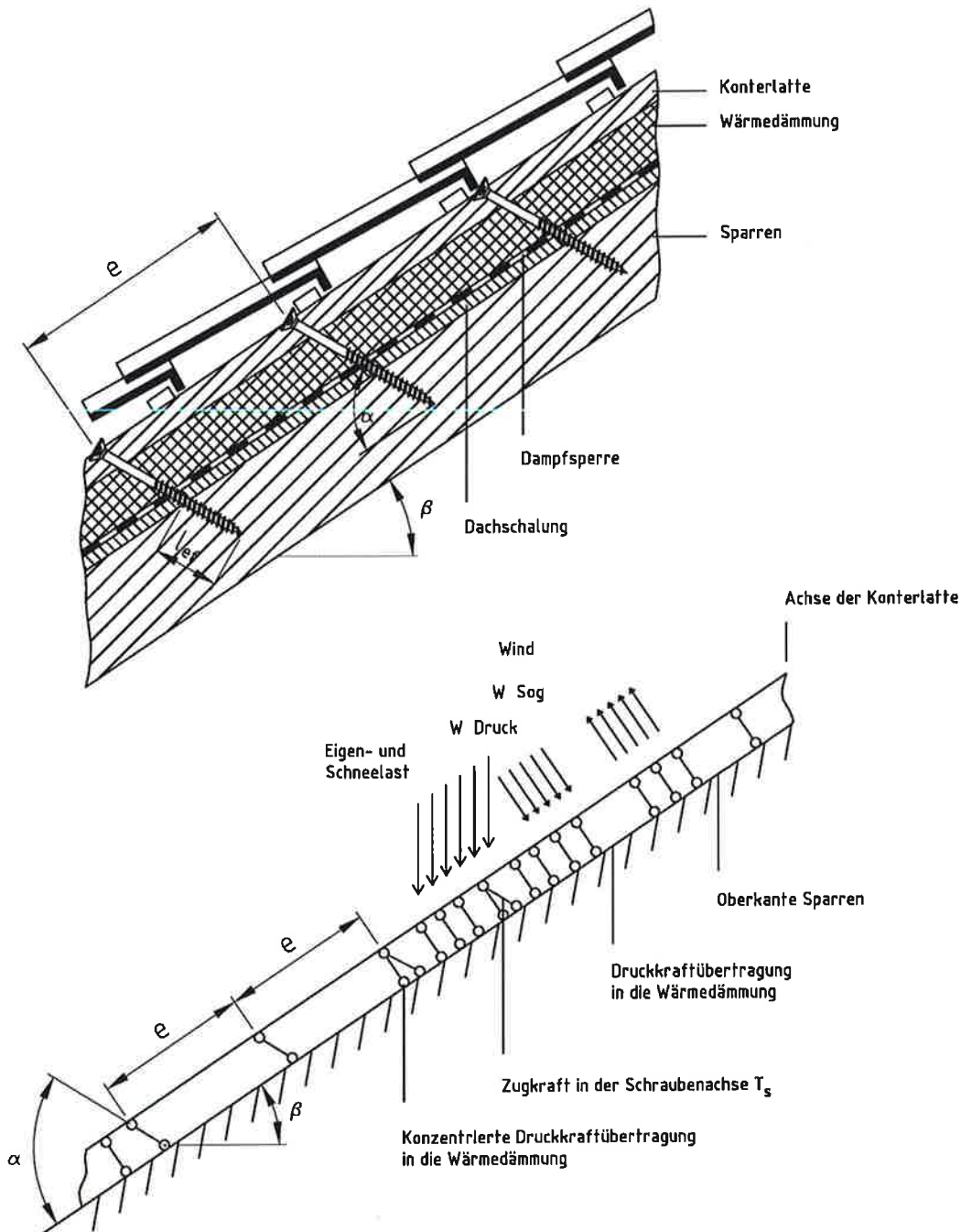
Abbildung 3.1: Befestigung von Aufdach-Dämmsystemen auf Sparren- Statisches Modell
